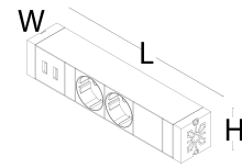
priz kutusu
